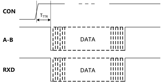
图 2. TDx01D485H-E模块数据接收时序图
