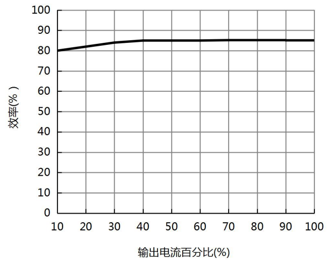
图 6. B0505S-1WR3效率vs输出负载(标称输入)
