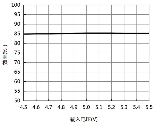
图 5. B0505LS-1WR3效率vs输入电压(满载)
