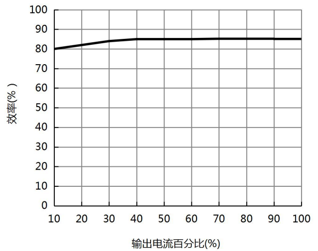
图 6. B0505LS-1WR3效率vs输出负载(标称输入)
